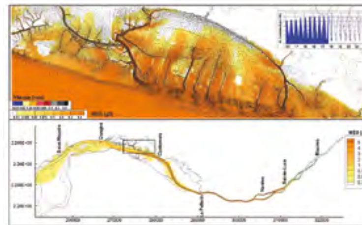
Figure 5 - Visualisation du débordement simulé le 17 septembre 2012: situation de pleine mer. Les vecteurs représentent le courant, tandis que la couleur du fond représente la concentration de matières en suspensions dans les secteurs inondés. La carte du haut est un zoom du secteur d'étude encadré dans la figure du bas, laquelle montre le positionnement du bouchon vaseux simulé.
