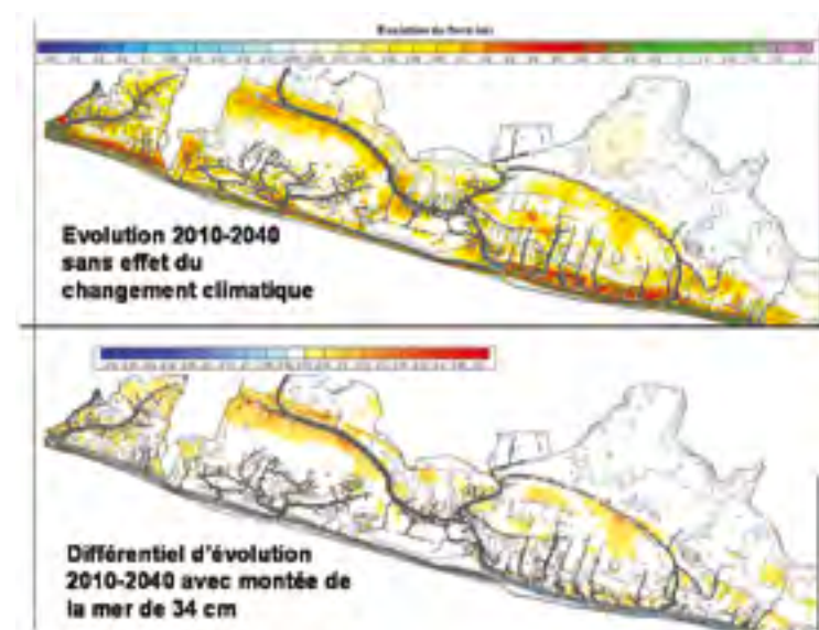
Figure 7 - Evolution topo-bathymétrique 2010-2040 pour le cas sans changement climatique et différentiel (avec ce cas) d'évolution pour le scénario de montée du niveau de la mer.
