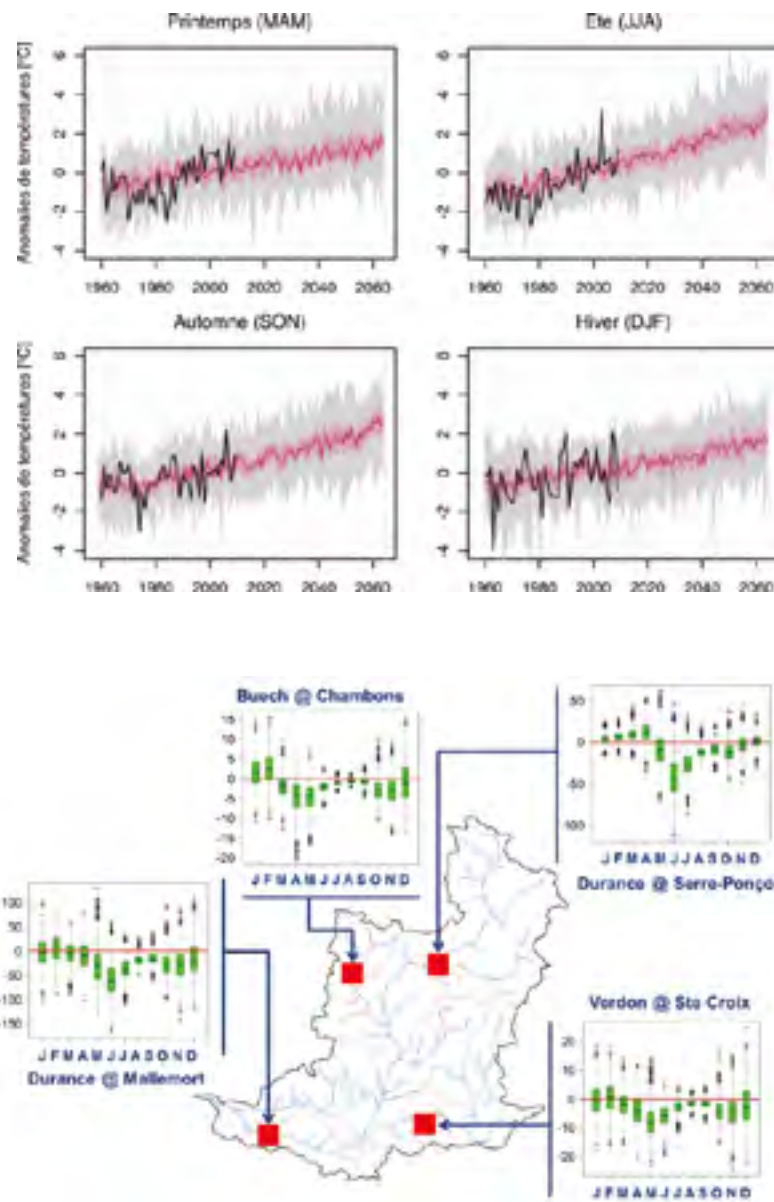
Figure 4 - Evolution des anomalies de températures saisonnières moyennes du bassin de la Durance à sa confluence avec le Rhône (en haut; les anomalies des 330 projections climatiques sont tracées en gris, la médiane est en rose foncé et l'enveloppe rose est l'intervalle entre les premiers et troisièmes quartiles; les forçages DuO sont représentés en noir) et les changements de débits mensuels exprimés en m³/s (en bas) sur la période 2036-2065, par rapport à la période de référence 1980-2009 (les boîtes sont définies par les premiers et troisièmes quartiles)
