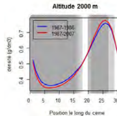
Figure 3 – Comparaison des profils moyens de cerne de mélèze formés à l'altitude 2000 m pendant la période 1967-1986 (plutôt fraîche) et pendant la période 1987-2007 (plutôt chaude). Le gris en arrière-plan indique les points du cerne pour lesquels les différences visibles sur le graphique sont significatives à 5% (gris clair), 1% (gris moyen) et 1/1000 (gris foncé).
