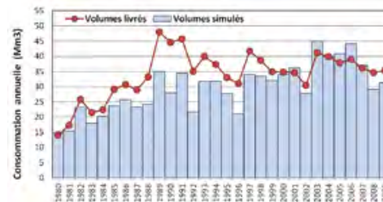
Figure 3 – Résultats de simulation des outils mobilisés dans R2D2 2050, en haut les débits décennaux moyens interannuels observés et simulés pour la Durance à Serre-Ponçon, en bas les consommations annuelles en eau d'irrigation simulées par le modèle FIVE-CoRe et livrées sur le périmètre desservi par la SCP
