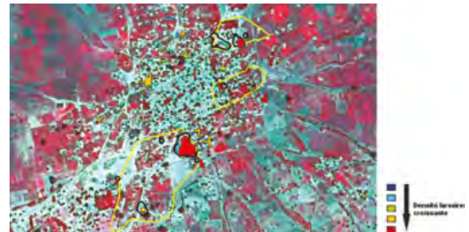
Figure 5 – Prédiction des densités larvaires d'anophèles
