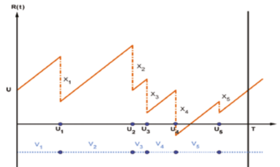
Figure 5 – Exemple de trajectoire du processus de réserve d'une compagnie d'assurance
