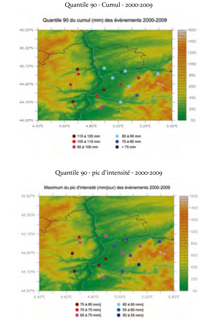
Figure 3 – Quantile 90 du cumul et du pic d'intensité des événements pluvieux enregistrés par les stations Météo-France (points de couleurs sur les cartes) au cours de la période 2000-2009 (définition CEMAGREF).
