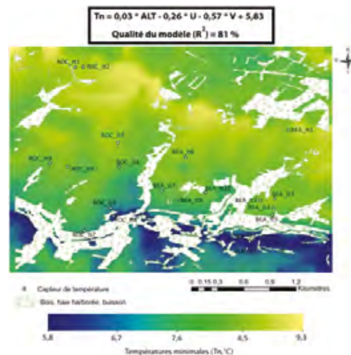
Figure 4: Spatialisation de la température minimale pour le mois d'octobre 2009 (Bonnefoy et al, 2014).
