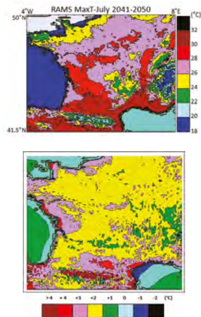
Figure 5 : Température maximale de juillet simulée par RAMS pour la période 2041-2050 sous conditions SRES A2 et pour la grille 2 (a) ; Différence entre 1991-2000 and 2041-2050 (b). (Bonnardot et al, 2012)
