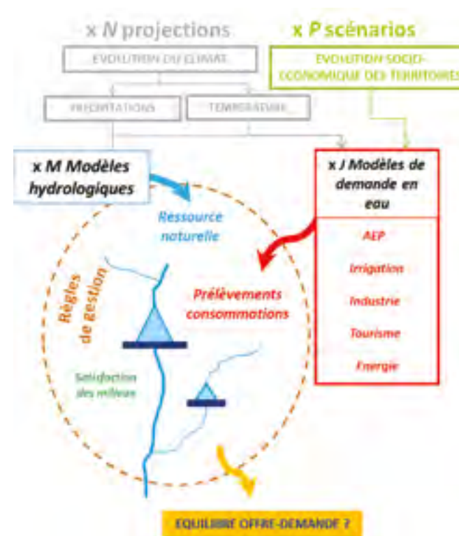
Figure 1 - Différentes composantes de la chaîne de modélisation
