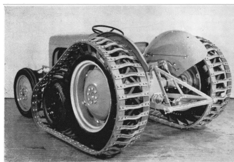
Fig. 4. Tracteur Ferguson équipé en semi-chenilles, Type « Bombardier ».
