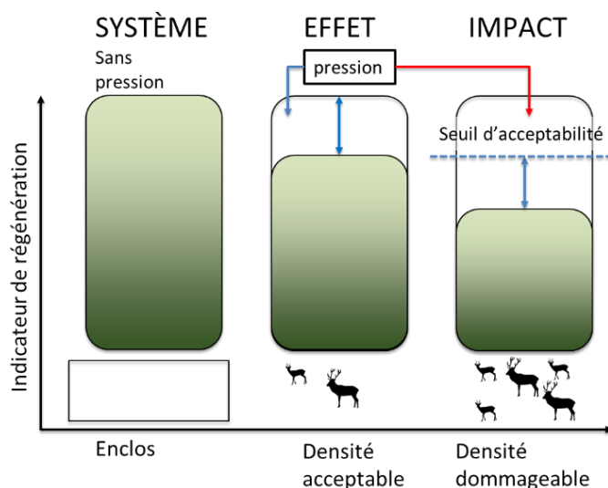
Figure 3.2-1 : Schéma fonctionnel des définitions des termes pression, effet et impact, d'après Mårell et al. (2015)
